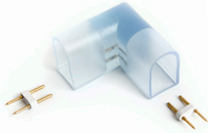
Соединитель угловой для ленты LS720, LS721
